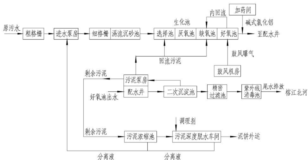
图 4-1 污水处理厂工艺流程图
