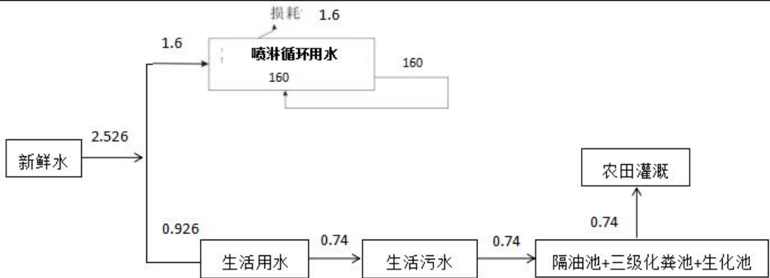
图 2-1 本项目水平衡图 (t/d)
