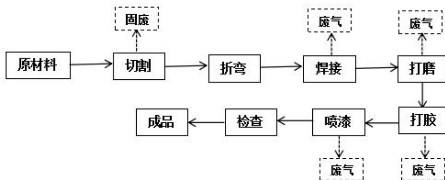
图 2-2 生产工艺流程图
