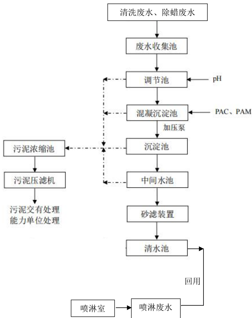
图 4.2-1 生产废水处理工艺流程
