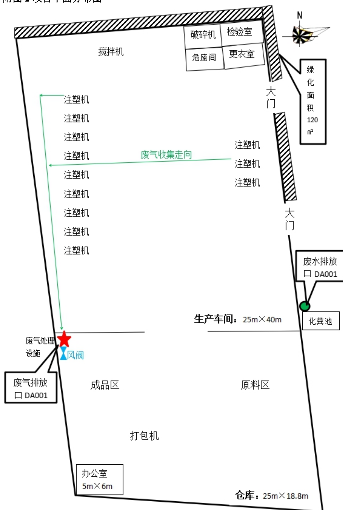
附图 2 项目平面分布图
