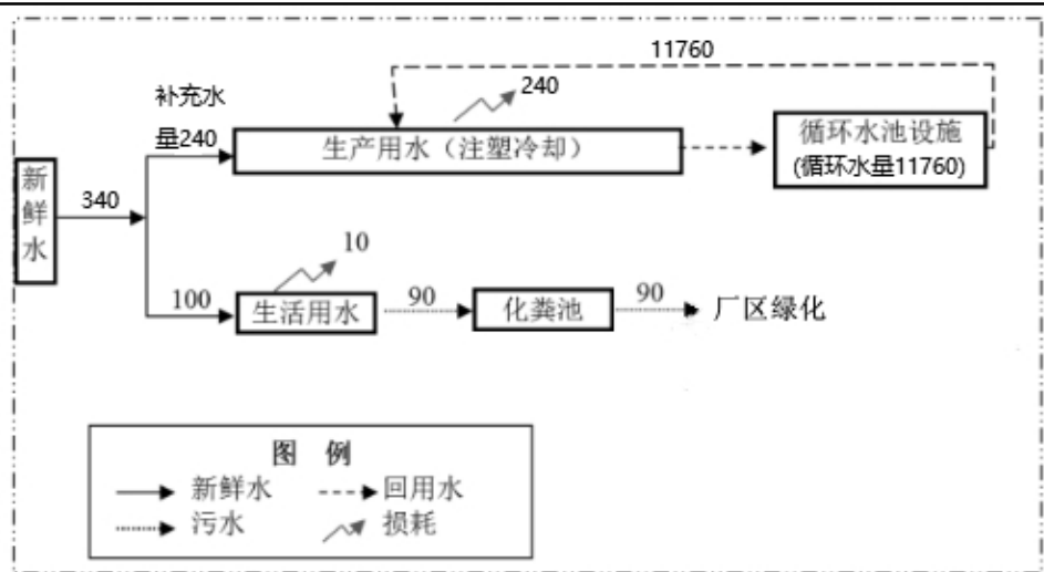
图 2-1 全厂用排水平衡图（单位：m³/a）
