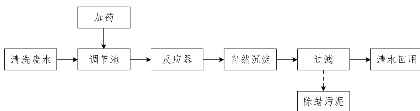
图 4-1 废水处理设施工艺流程
