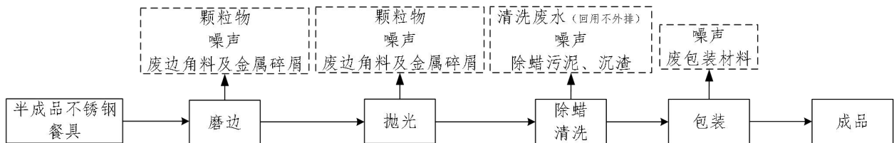
图 2-2 不锈钢餐具生产加工处理工艺流程图
