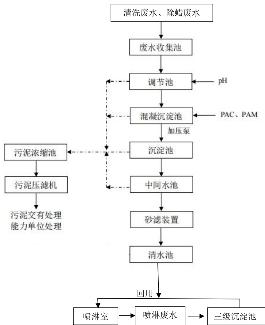
图 4.2-1 生产废水处理工艺流程
