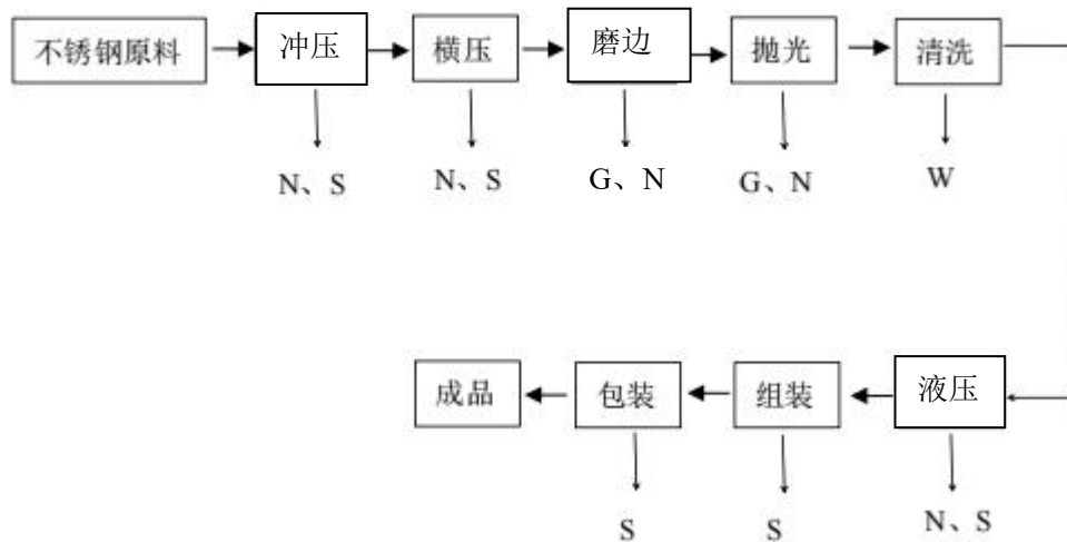
图 2-2 半成品五金件工艺流程图
