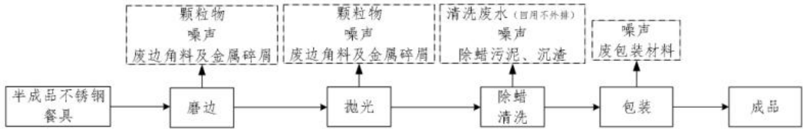
图 2-2 生产工艺流程及产排污环节图
