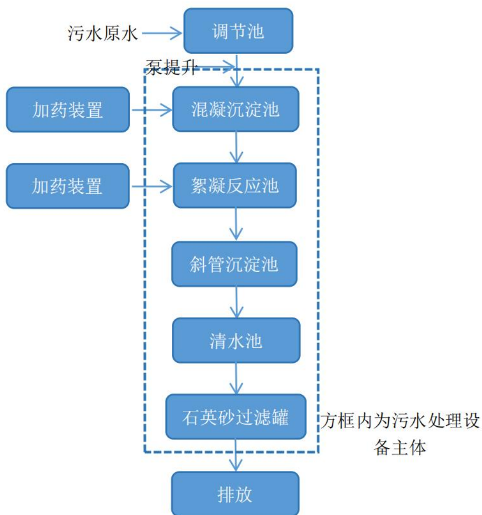
图 4-1 清洗废水处理工艺流程图
