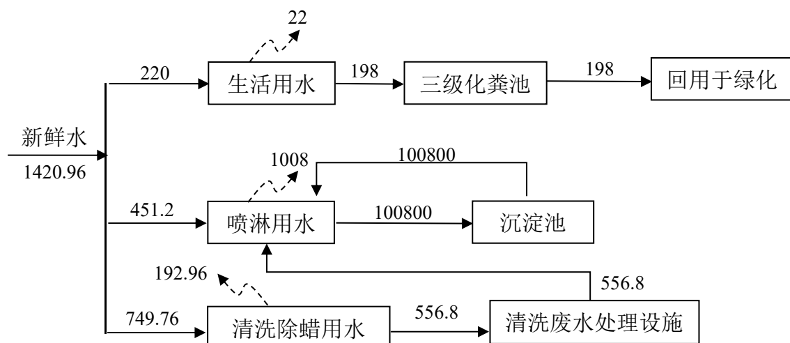
图 2-1 项目总体水平衡图 (单位: m³/a)
