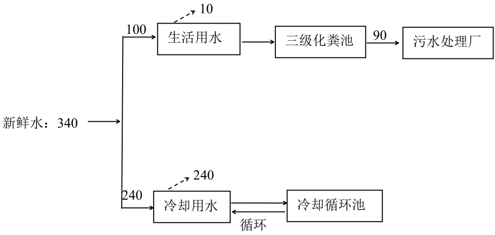
图 2-1 全厂用排水平衡图（单位：m³/a）
