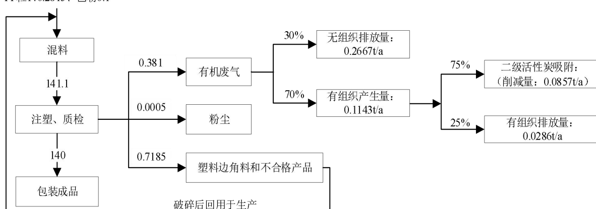
图 2-1 项目物料平衡图 (t/a)
