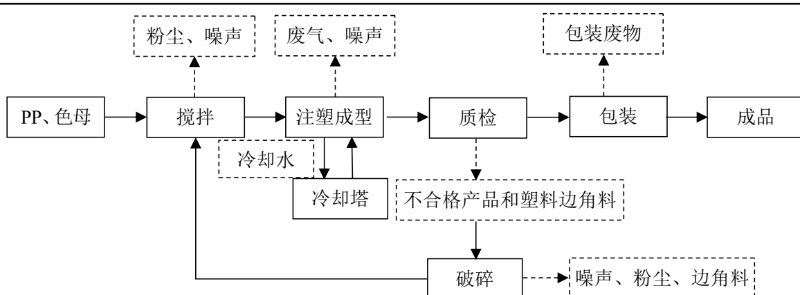
图 2-3 项目生产工艺流程及产污环节
