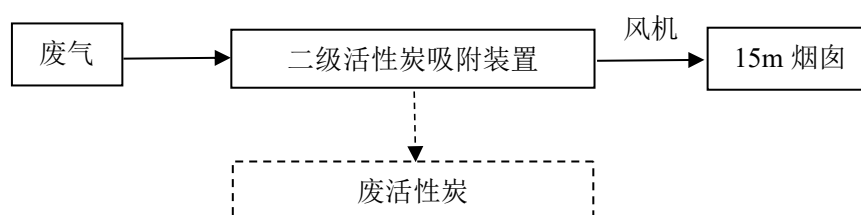
图 2-4 项目废气流程及产污环节
