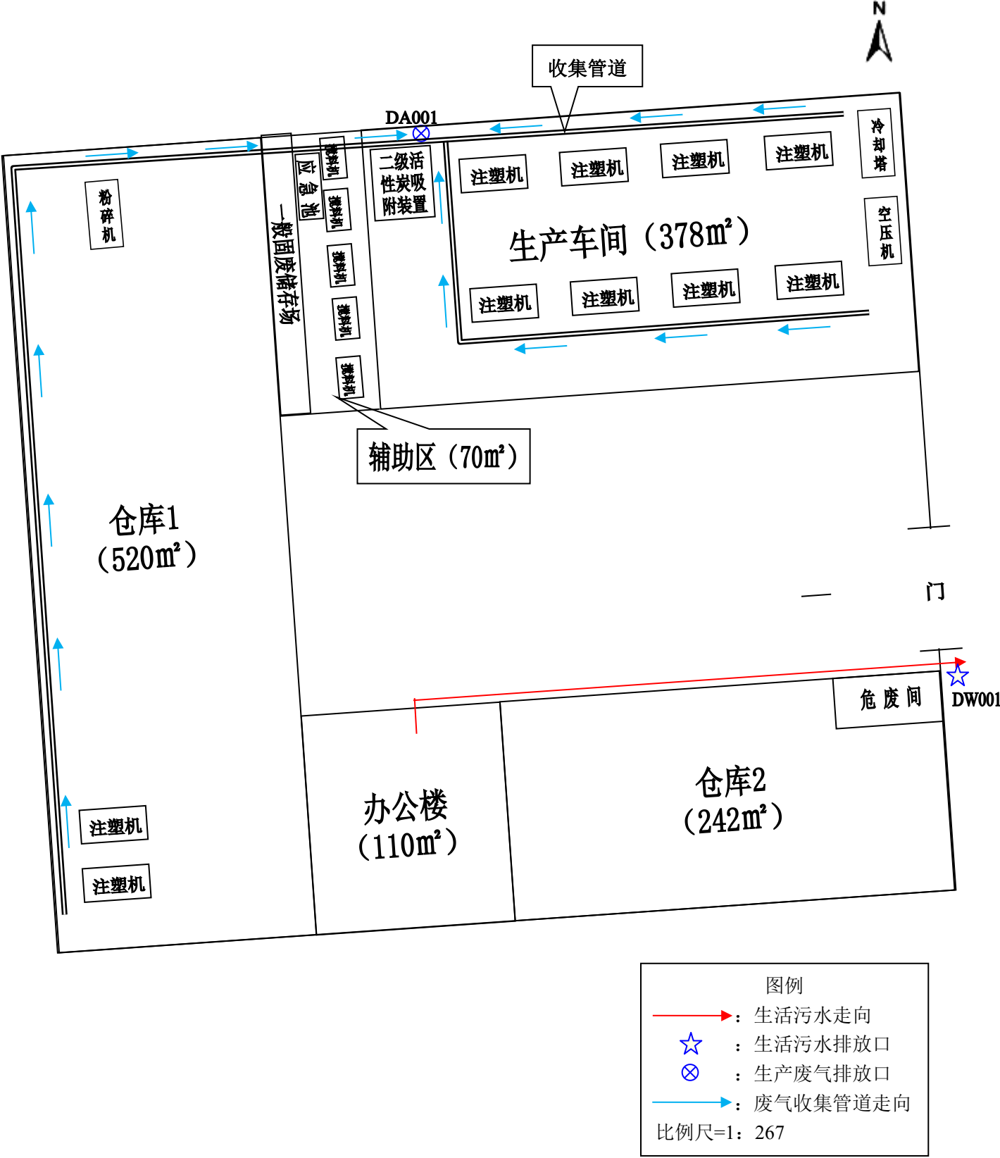
附图 5：项目平面布置图
