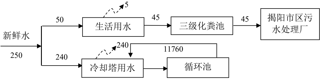
图 2-2 项目建成后全厂用水平衡图（单位：t/a）
