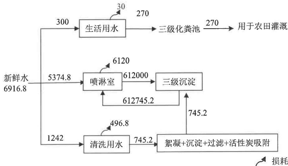
图 2-1 项目总用水平衡图 单位：m³/a
