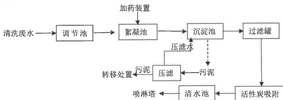
图 4-1 清洗废水处理工艺流程
