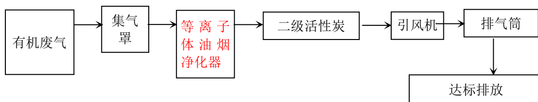
图 4-1 项目废气处理工艺流程图
