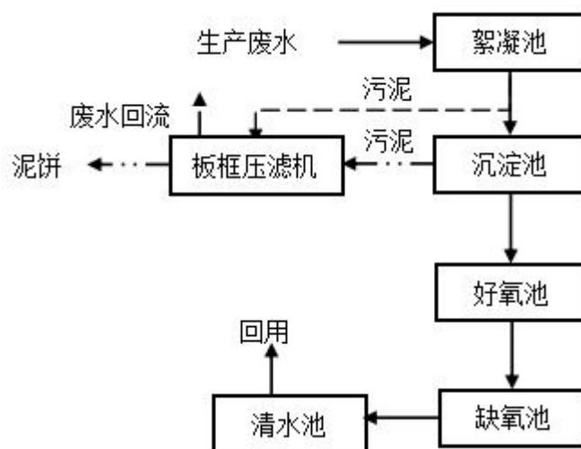
图 4-3 废水处理工艺流程图
