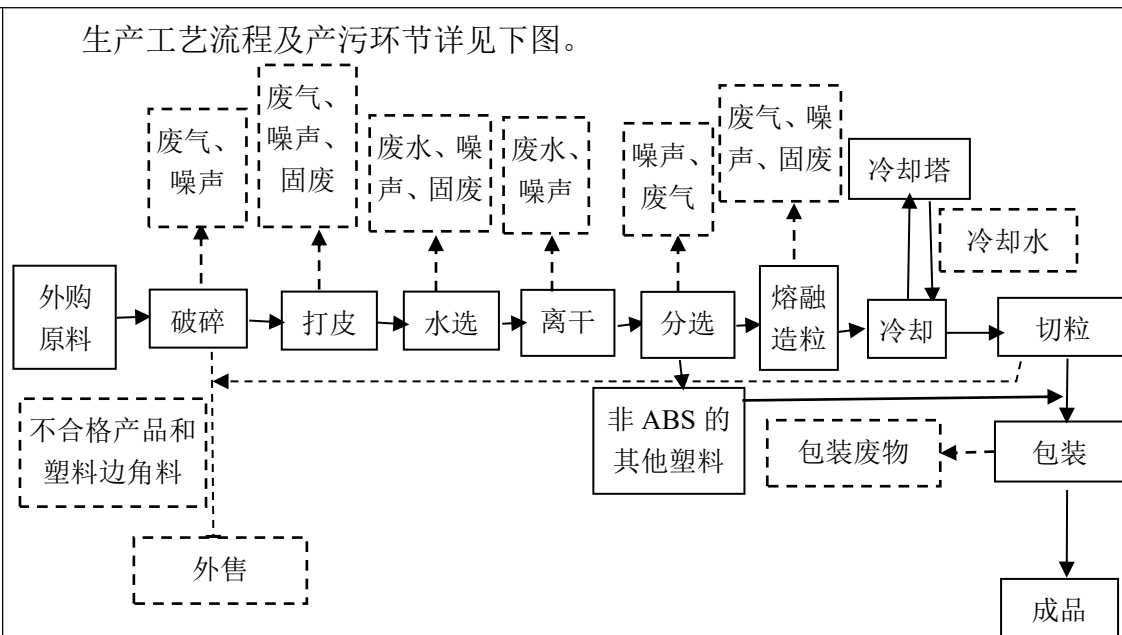
图 2-2 项目生产工艺流程及产污环节
