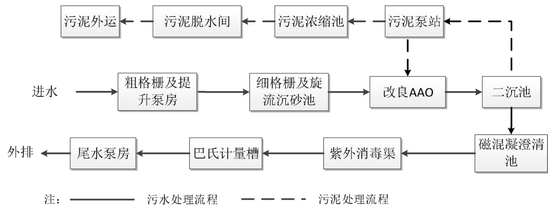
图 4.2-1 揭阳市榕城区北部水质净化厂工艺流程图
