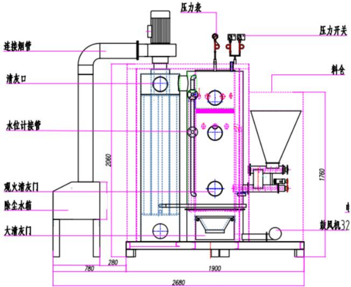
图4-1 生物质蒸汽炉结构图
