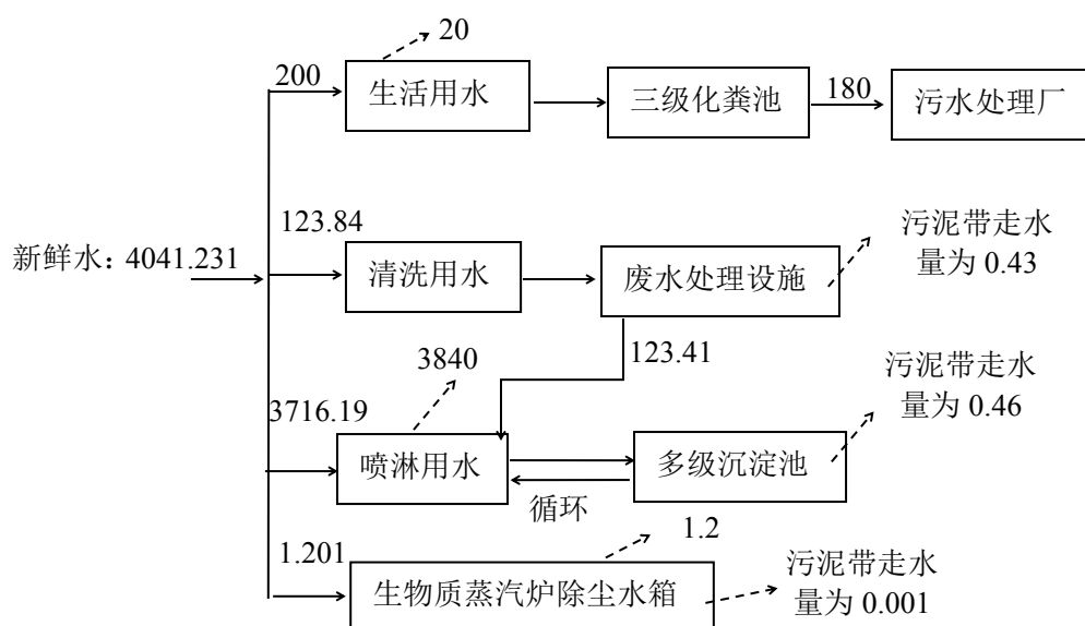
图 4-6 全厂用排水平衡图 (m³/a)
