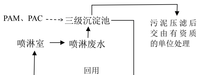
图 4-4 喷淋废水处理工艺流程
