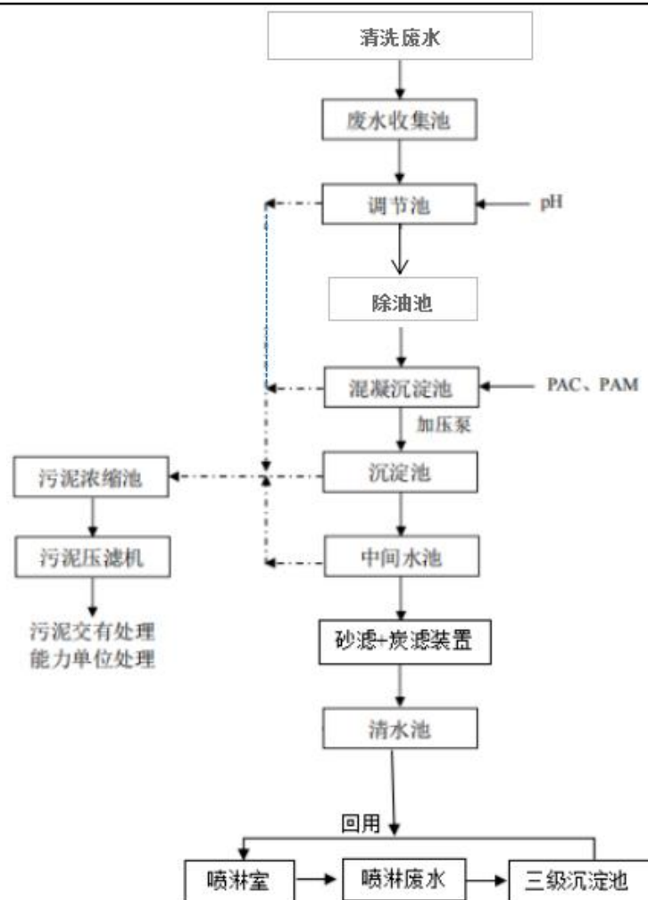
图 4-3 生产废水处理工艺流程
