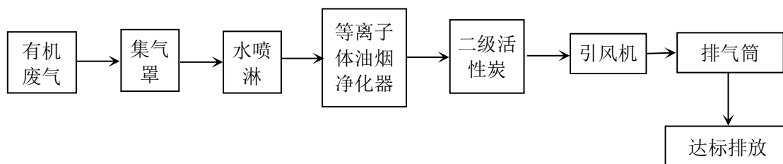
图 4-1 项目废气处理工艺流程图
