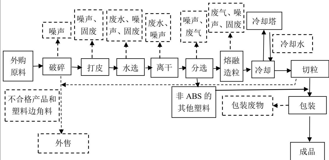
图 2-2 项目生产工艺流程及产污环节
