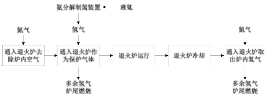
图 2-5 退火工艺流程及产污环节图
