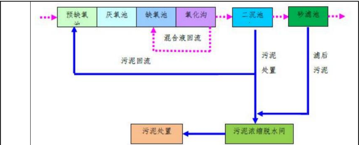
图 4-3 污水处理工艺流程图
