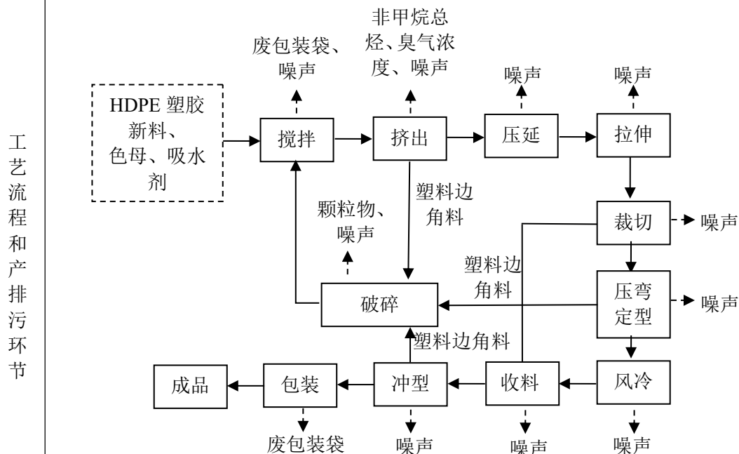
图 2-2 工艺流程图
