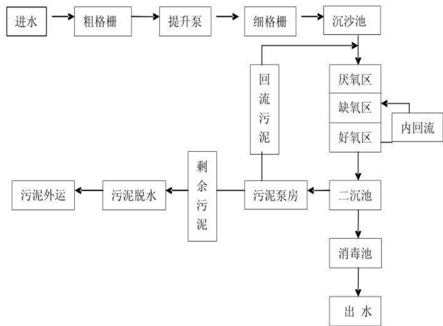
图 4-1 揭阳市区污水处理厂工艺流程图
