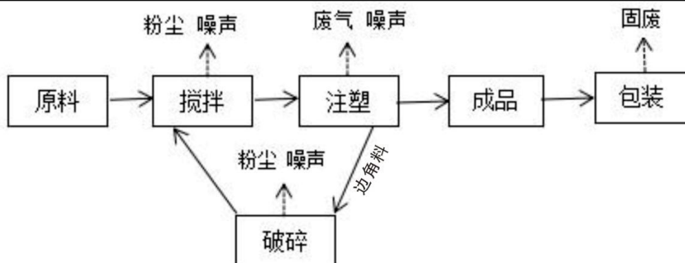
图 2-2 工艺流程图
