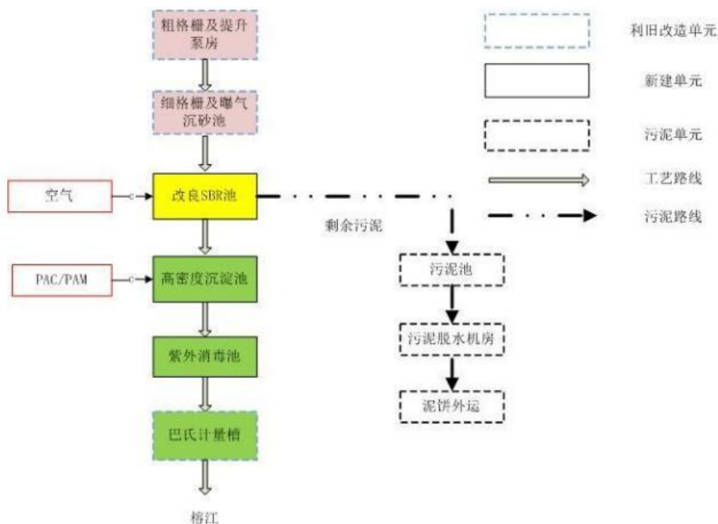
图 4-2 揭阳原空港经济区污水处理厂扩建及配套管网建设工程工艺流程图 揭阳空港经济区污水处理厂设计进出水水质标准见下表。
