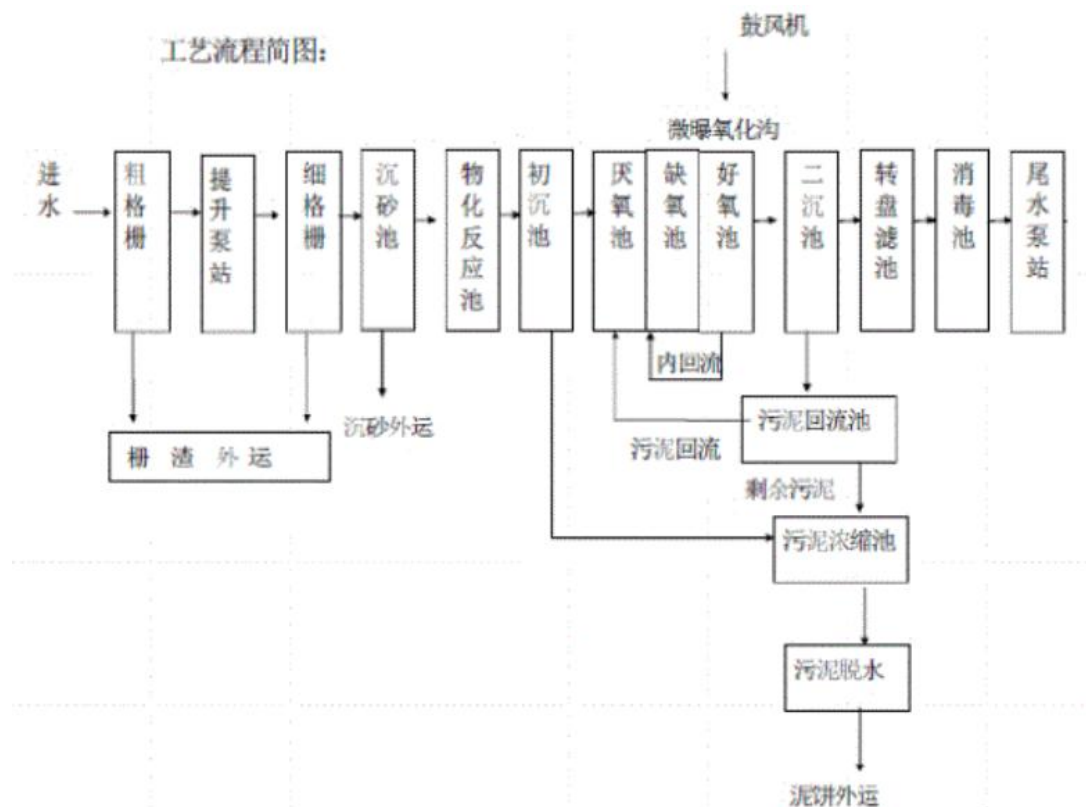
图 4-1 揭阳空港经济区污水处理厂（近期）工艺流程图
