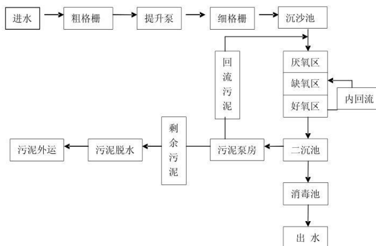
图 4-1 揭阳市区污水处理厂工艺流程图
