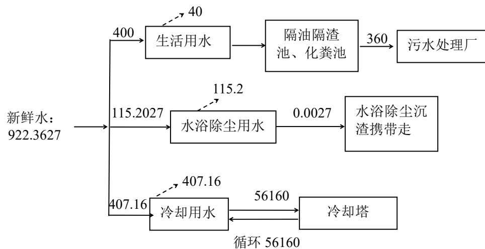
图 2-1 全厂用排水平衡图（单位：m³/a）
