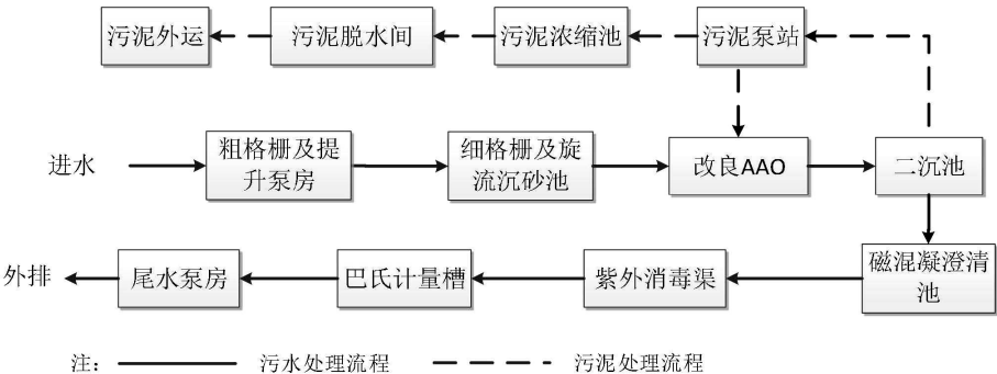
图 4-1 揭阳市榕城区中部水质净化厂工艺流程图
