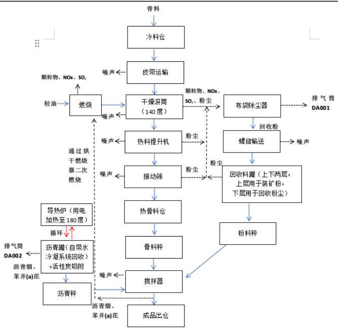
图 2-2 项目工艺流程图
