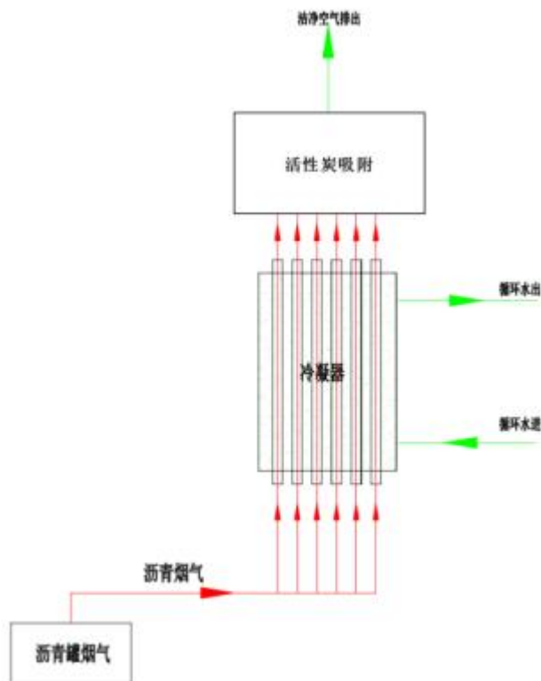
图 4-1 沥青烟气处理流程图
