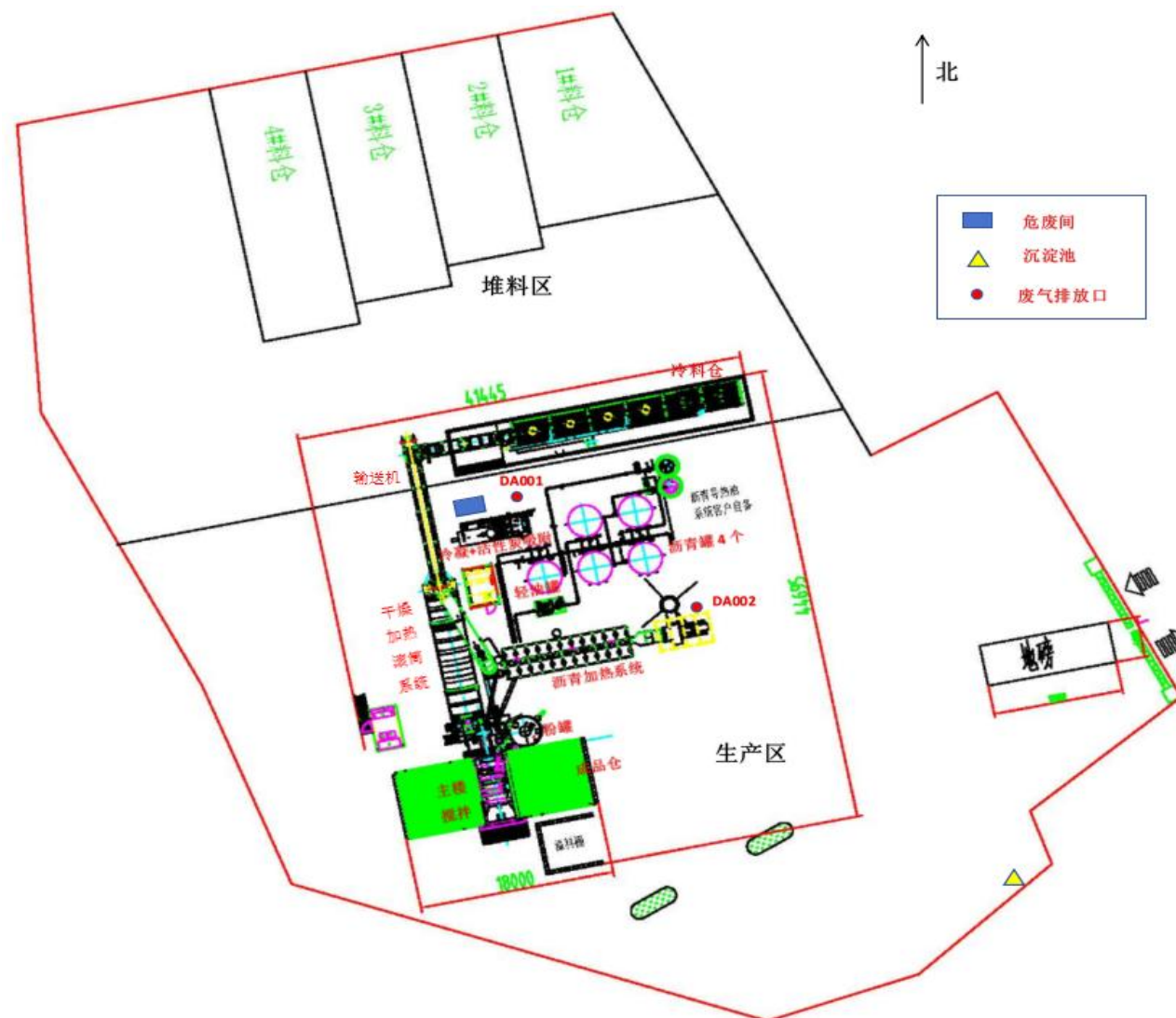
附图 4 项目平面图
