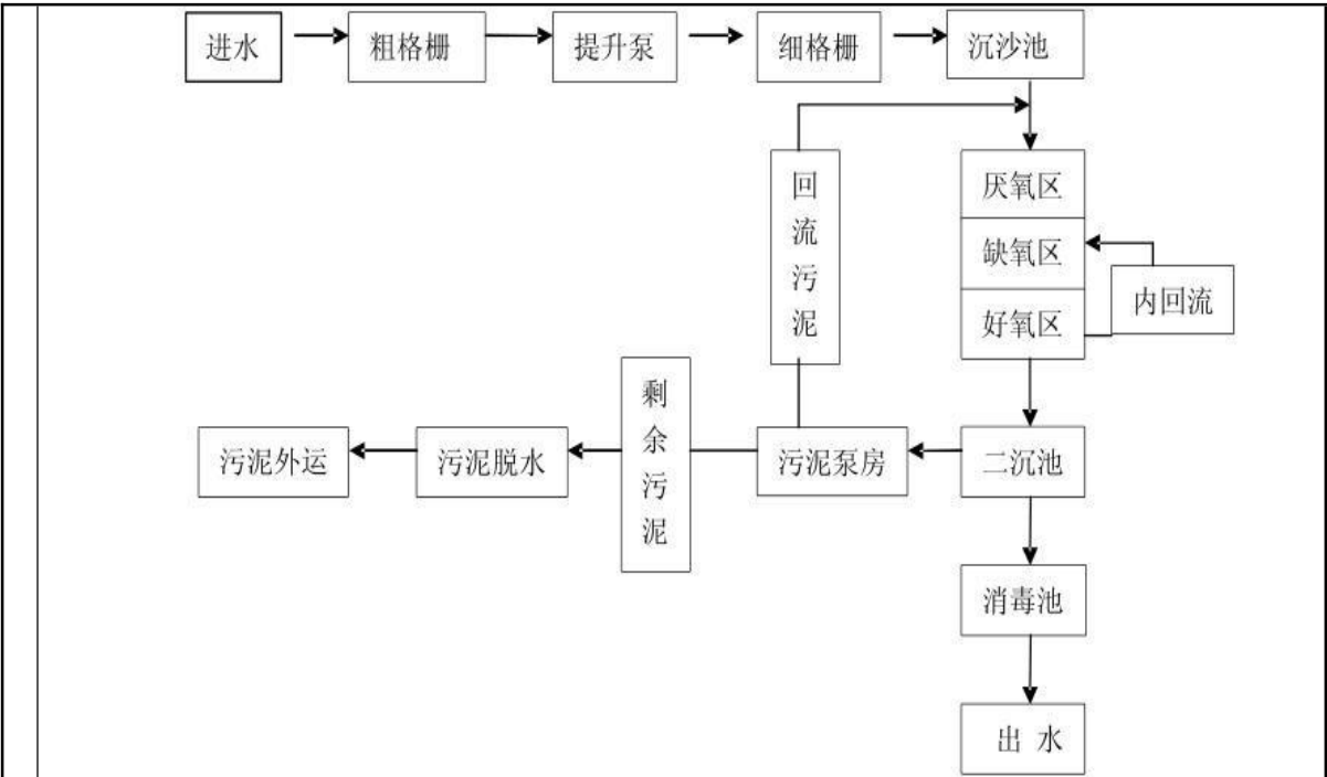
图 4.2-1 揭阳市区污水处理厂工艺流程图
