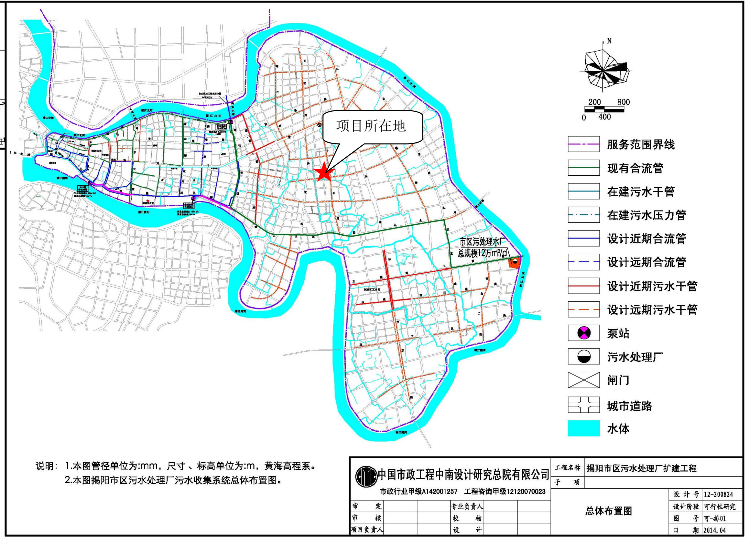
附图 9 揭阳市区污水处理厂管网图
