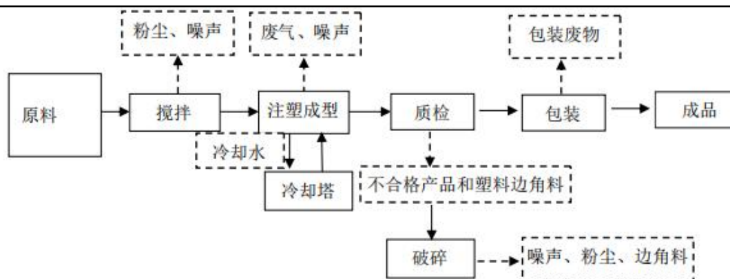
图 2-2 工艺流程图
