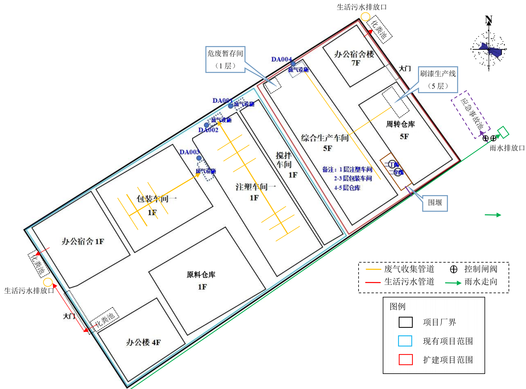
附图 5 项目总平面布置图
