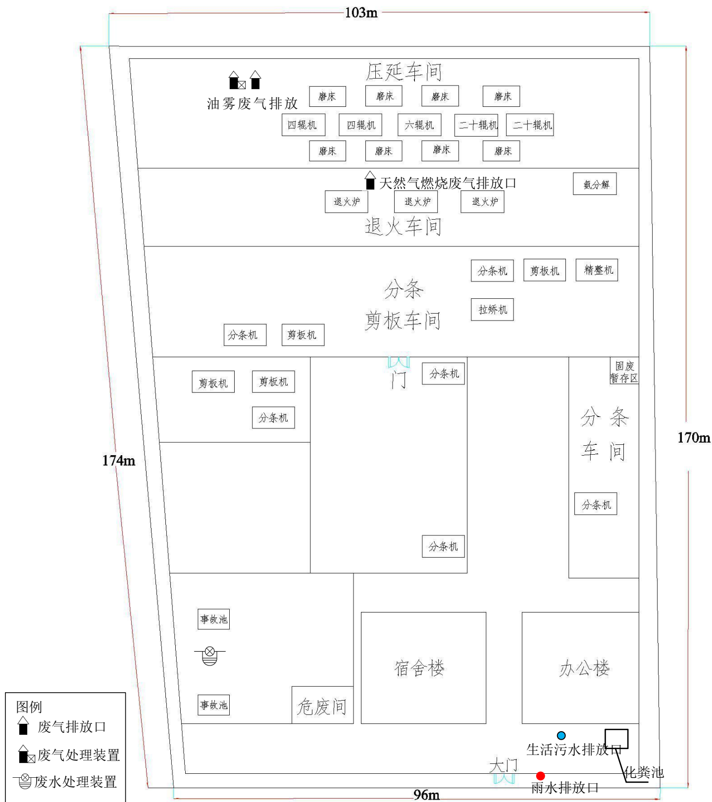
附图 3 项目平面布置图
