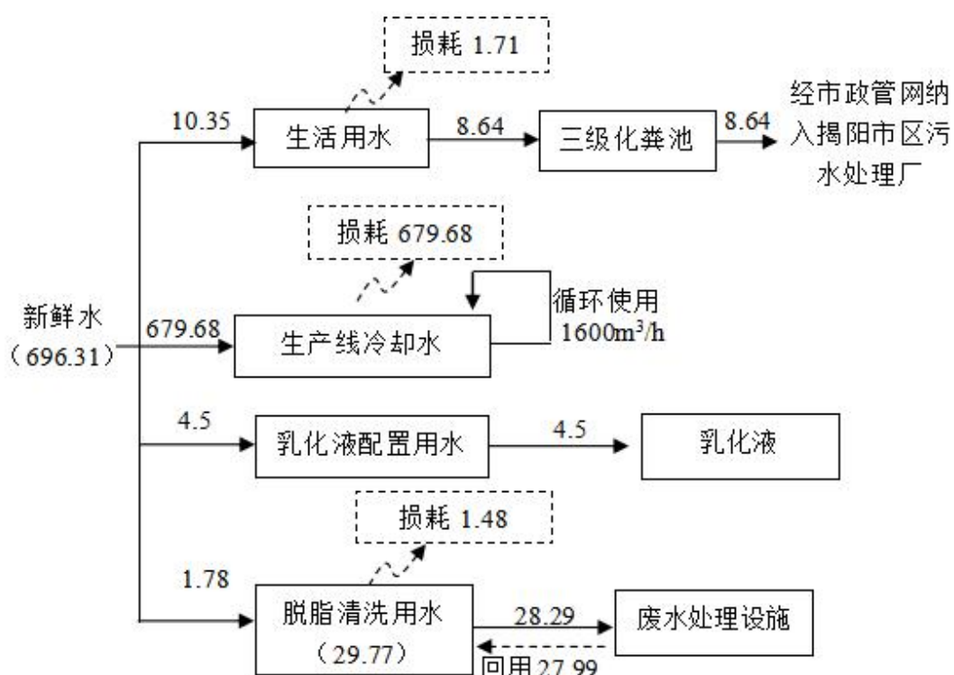
图 2-1 改扩建项目建成后全厂水平衡图 单位：t/d
