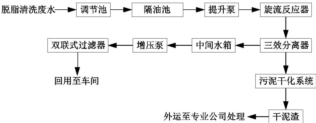
图 4-1 依托的废水处理工艺流程图
