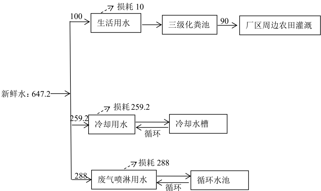
图 2-2 项目水平衡图（单位：m 3 /a）
