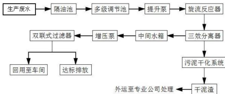
图 2-6 原项目生产流程图及产污环节
