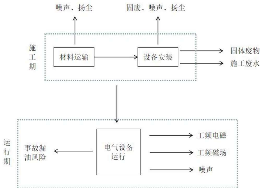
图 2-4 工艺流程及产污环节图
