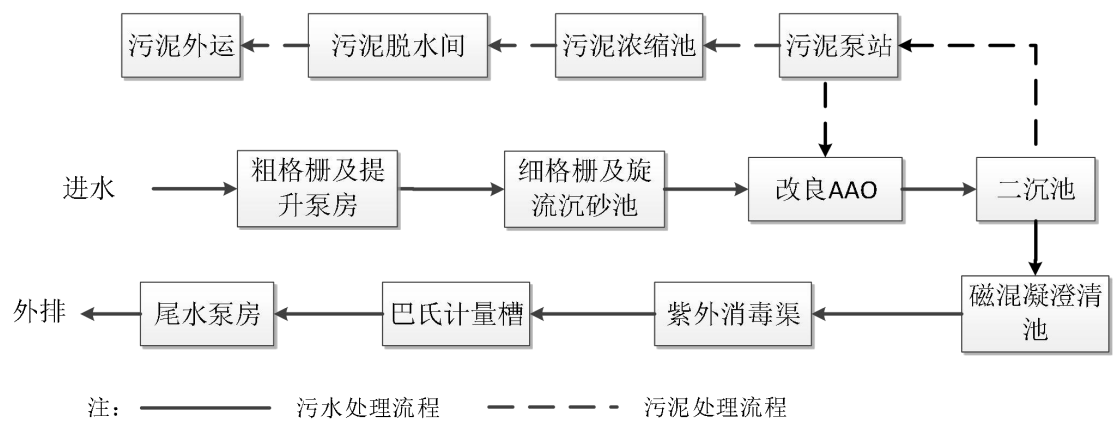
图 4-3 揭阳市榕城区北部水质净化厂工艺流程图
