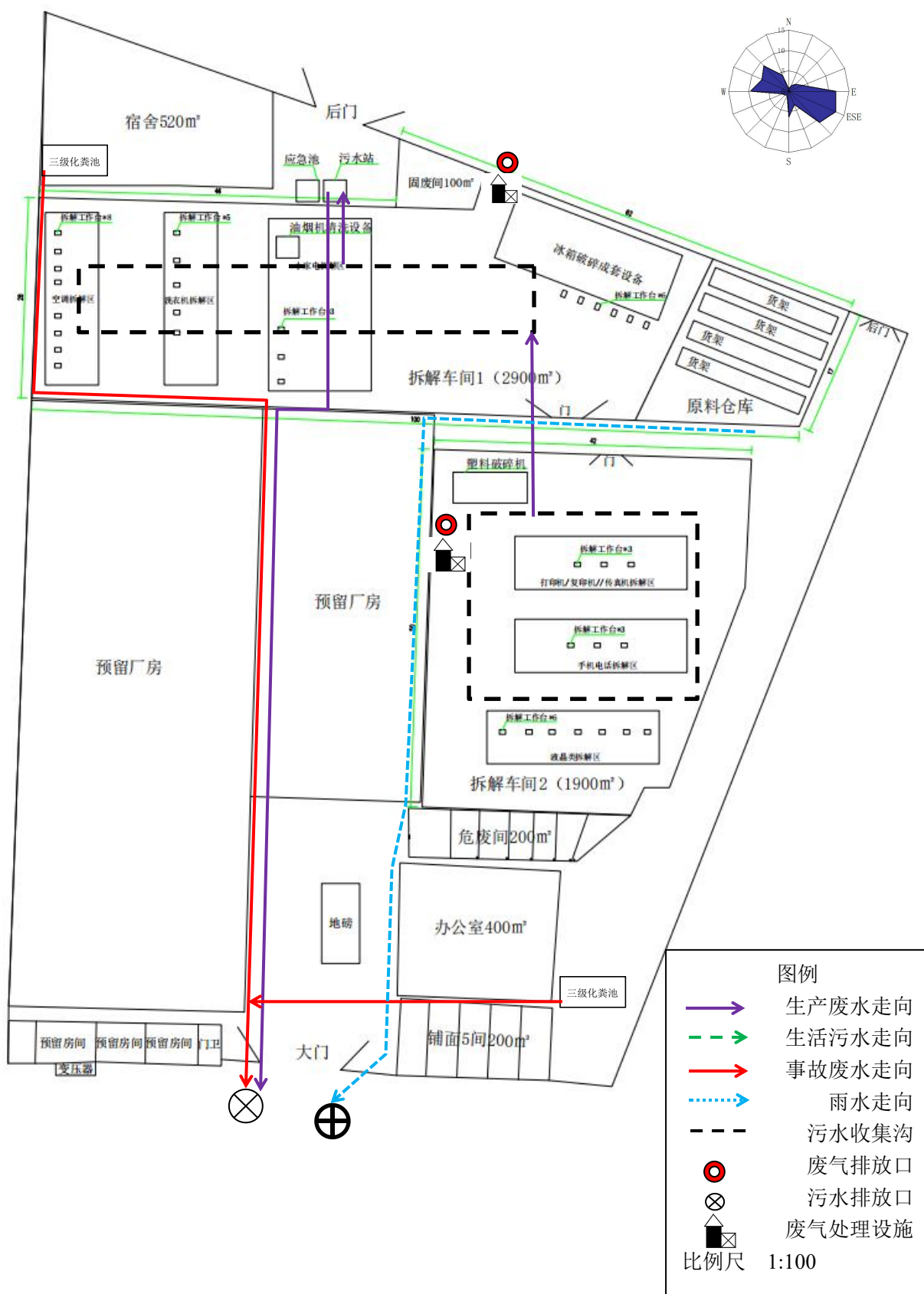
附图 4 项目总平面图
