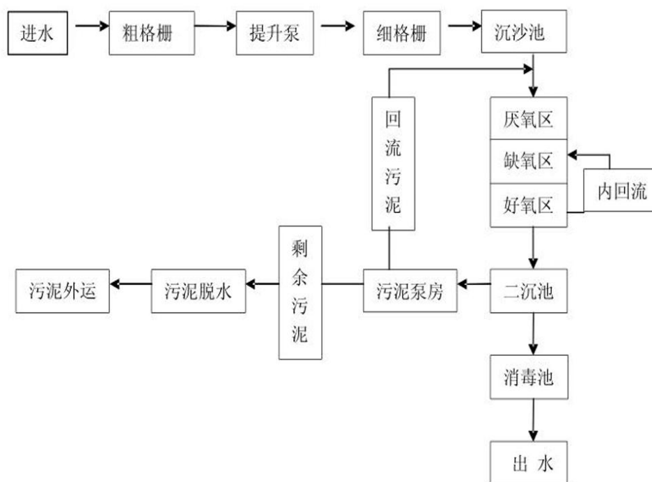
图 4-1 揭阳市榕城区仙梅污水处理厂污水处理工艺流程图
