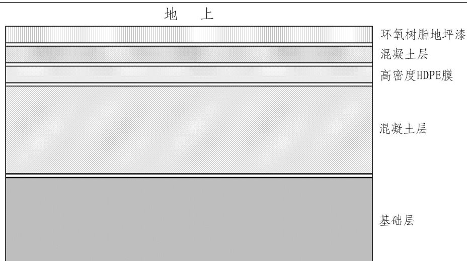
图 2-1 项目拟设置防渗层结构示意图
