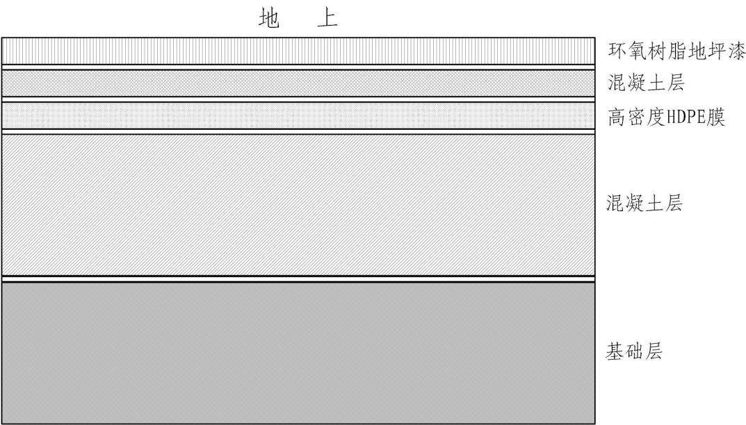
图 4-3 项目防渗层结构示意图
