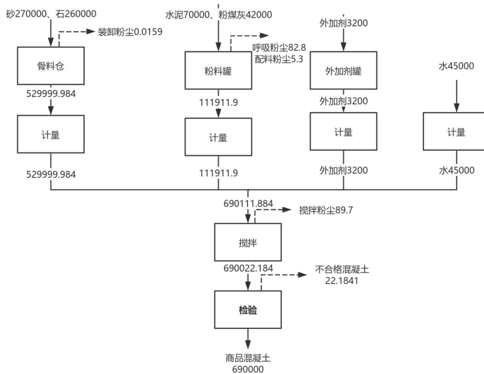
图 2-2 项目物料平衡图 (t/a)
