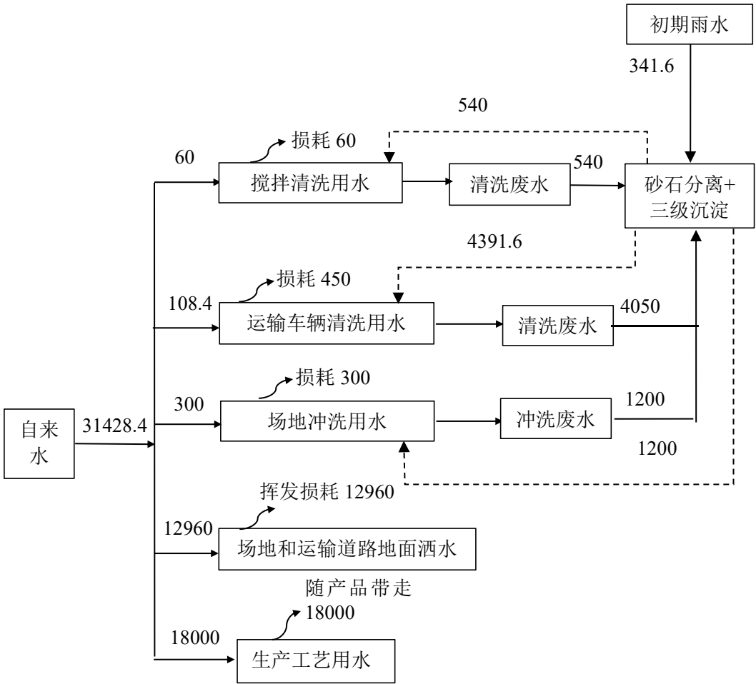
图1 扩建项目水平衡图 单位：m³/a
