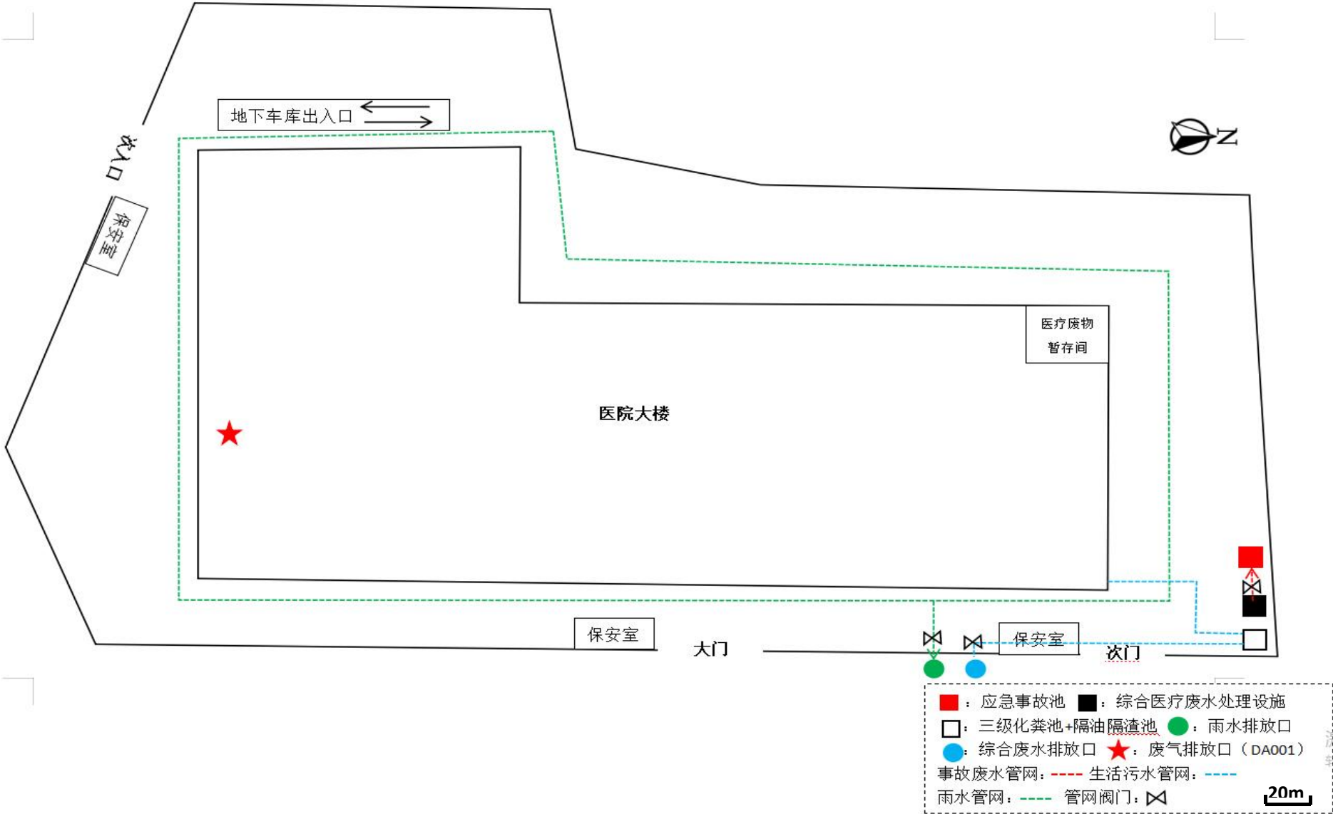
附图 3-1 项目总平面布置
