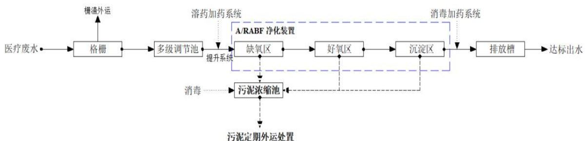
图 4-1 废水处理设施工艺流程
