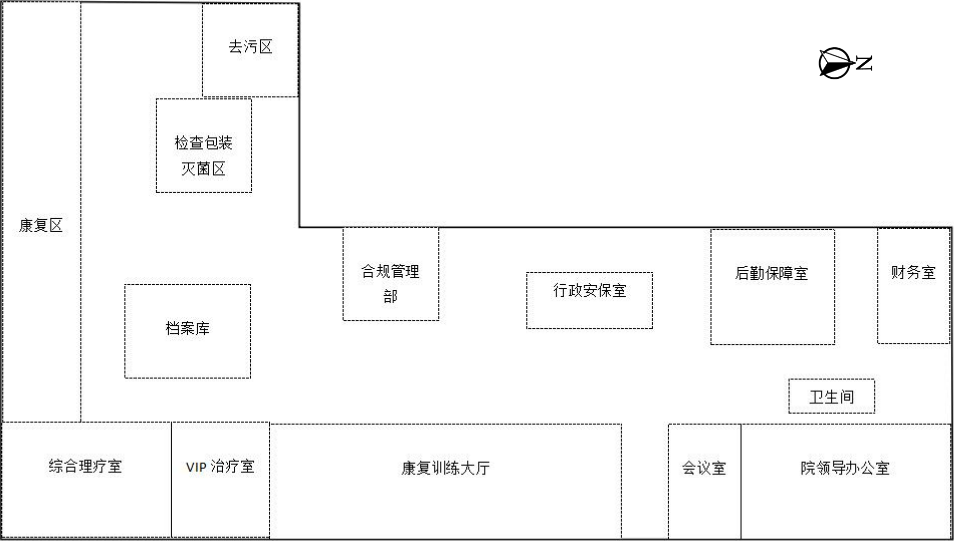
附图 3-4 项目主楼 3 层平面布置图
