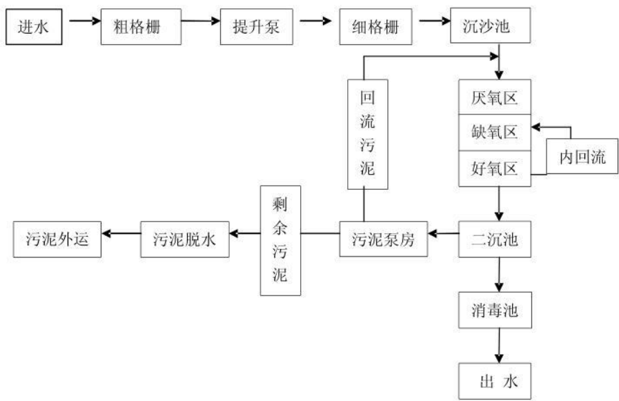
图 4-3 仙梅污水处理厂工艺流程图
