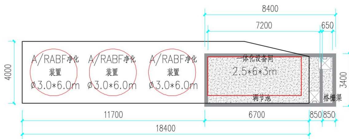
图 4-2 废水处理设施平面布置图
