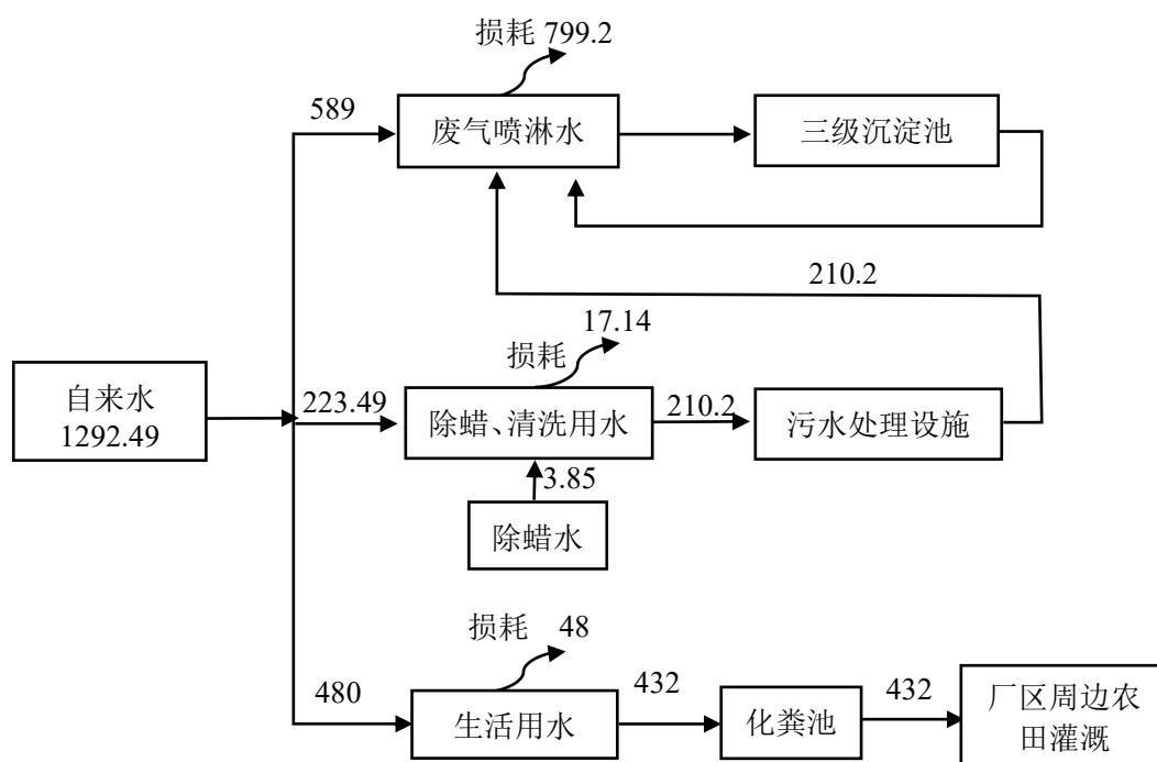
图 2-1 项目全厂区水平衡图（ \text{m}^3/\text{a} ）
