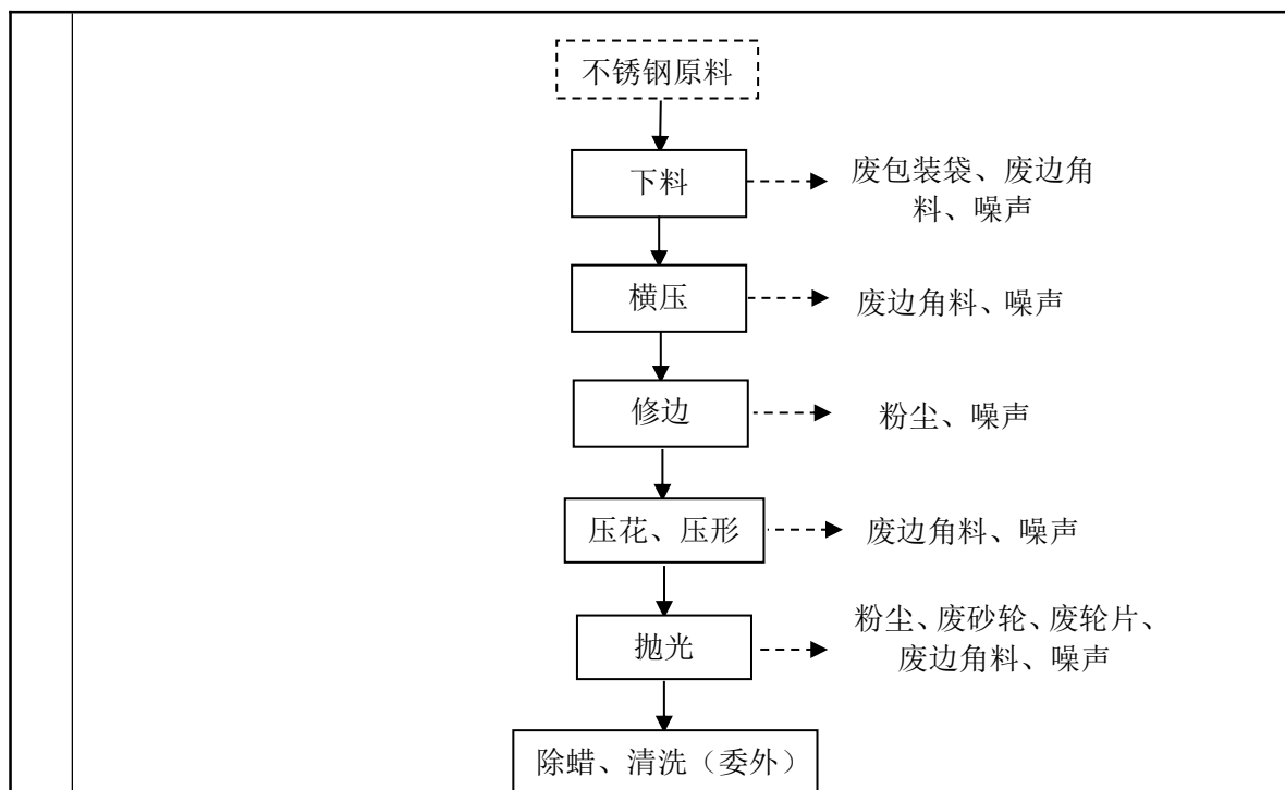
图 2-2 扩建前项目不锈钢餐具生产工艺流程
