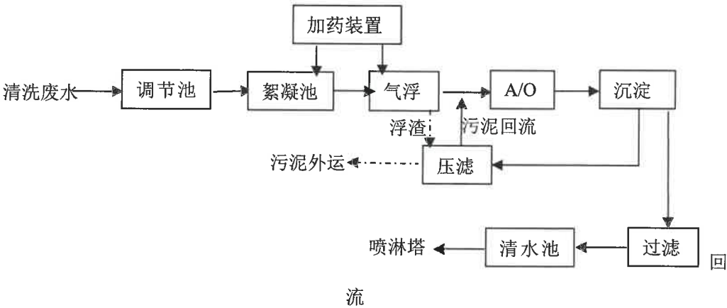
图 4-1 清洗废水处理工艺流程
