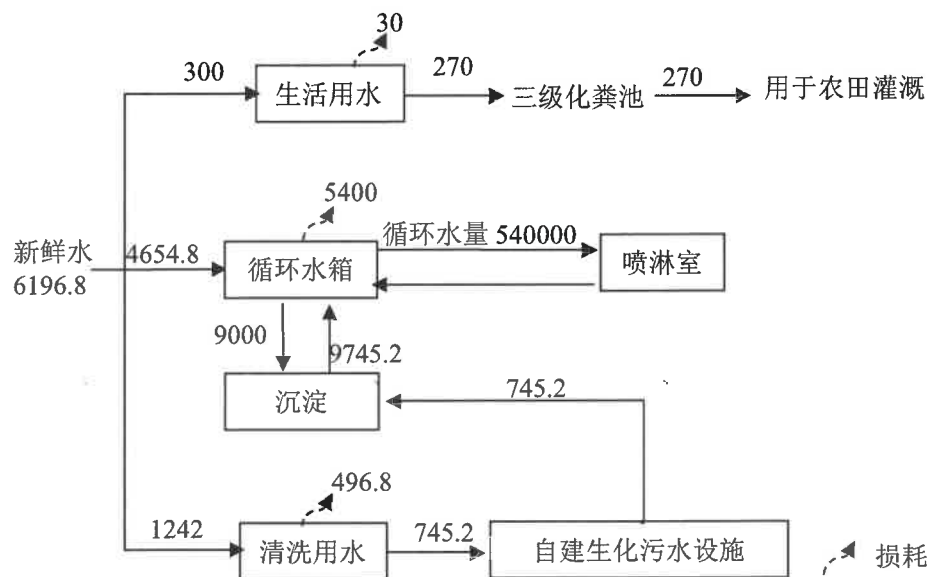
图 2-1 项目总用水平衡图 单位: \text{m}^3/\text{a}
