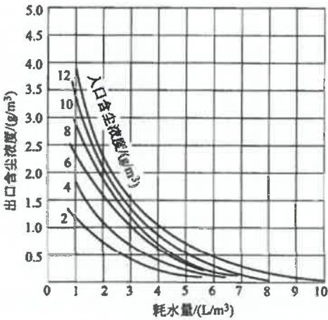
图 5-49 空心喷雾洗涤除尘器 净化炉煤气粉尘耗水量与 进出口气体中含尘浓度的关系
