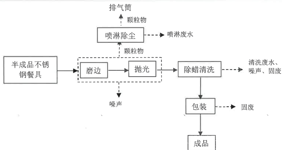
图 2-1 不锈钢餐具加工工艺流程及产污节点图
